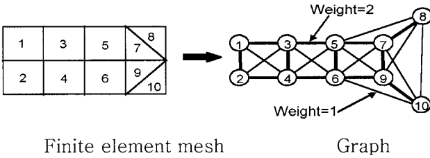
Fig. 4 WEM scheme.
